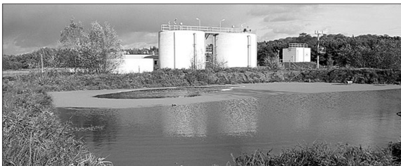
Ryc. 13. Grotniki – gminna oczyszczalnia ścieków o wydajno- ści 740 m 3 na dobę, zbudowana w 1997 r.
