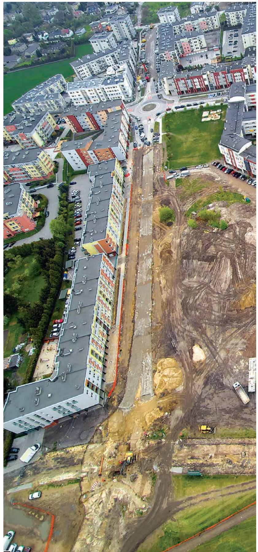
Zdjęcie wykonane z lotu ptaka – na 1. planie, u dołu, trwają prace przy budowie ronda na skrzyżowaniu al. Jana Pawła II z ul. Pułaskiego. Dalej, w górę, widzimy częściowo wykonany chodnik po stronie bloków z adresem: al. Jana Pawła II 7 i 9 oraz koryto przyszłej jezdni; następnie gotowe rondo na ul. Wschodniej (wykonane w ub. roku). Kolejny odcinek – w kierunku ul. Konarzewskiego – na którym trzeba wykonać dodatkowo oświetlenie uliczne (zastawiony jeszcze przez urządzenia budujące blok przy ul. Wschodniej 26) fot. Rafał Wojtyniak
